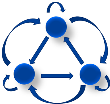
图 2. 状态转移
